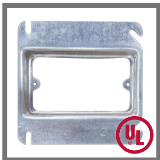
TAPA PARA CAJA CUADRADA EMT CON ORIFICIO RECTANGULAR
