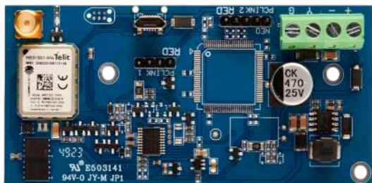
COMUNICADOR CELULAR ESIM DUAL SIM 5G LTE
